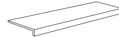
LCPE609R Lago di Como Perla LCSA609R Lago di Como Sabbia LCCE609R Lago di Como Cenere LCGR609R Lago di Como Grafite Gradino a L. costa retta lineare cm 30x120x5h - 11 3/4" x 48" x 2" Rettificato sp. 9,5 mm
