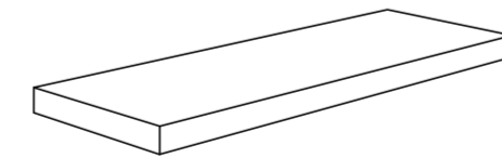
LCPE612R Lago di Como Perla LCSA612R Lago di Como Sabbia LCCE612R Lago di Como Cenere LCGR612R Lago di Como Grafite Gradino angolare costa retta lineare (vers. A) cm 30x120x5h - 11 3/4" x 48" x 2" Rettificato sp. 9,5 mm
